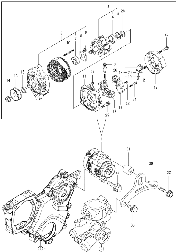
0CW10-M47000 3TNM68-HGEP Fig.17. (15A)GENERATOR
